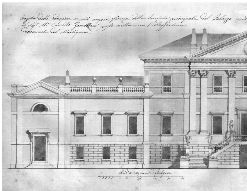
Progetto facciata Palazzo Zambeccari in località Martignone.
