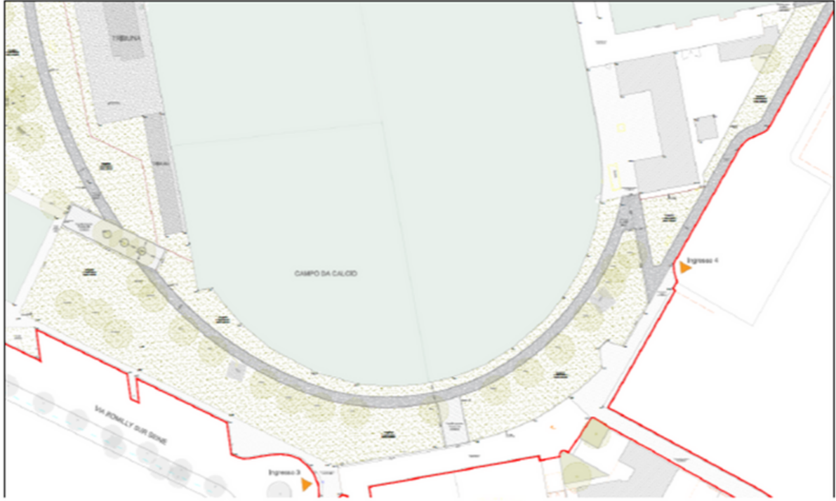
Stralcio Planimetria Stato Futuro Area perimetrale allo stadio
