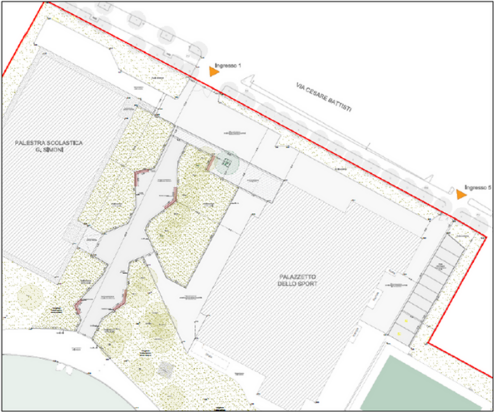
Stralcio Planimetria Stato Futuro Area di Accesso 01
